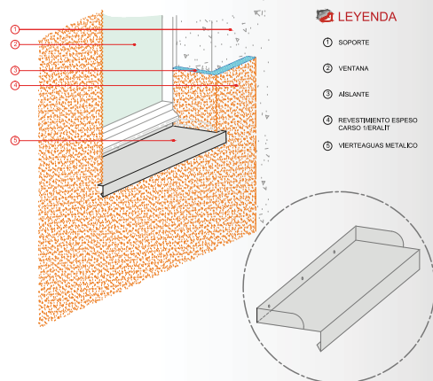
DETALLE 12
