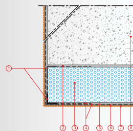
CORTE HORIZONTAL
