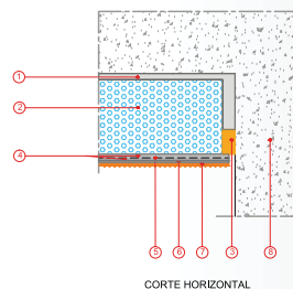
CORTE HORIZONTAL
