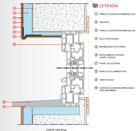
DETALLE 11
