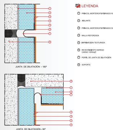
DETALLE 13
